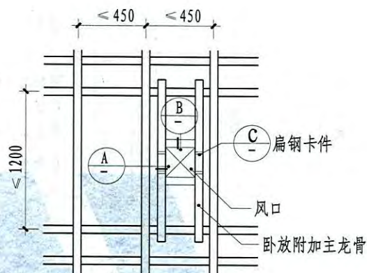
2 (风口不影响吊顶龙骨)
