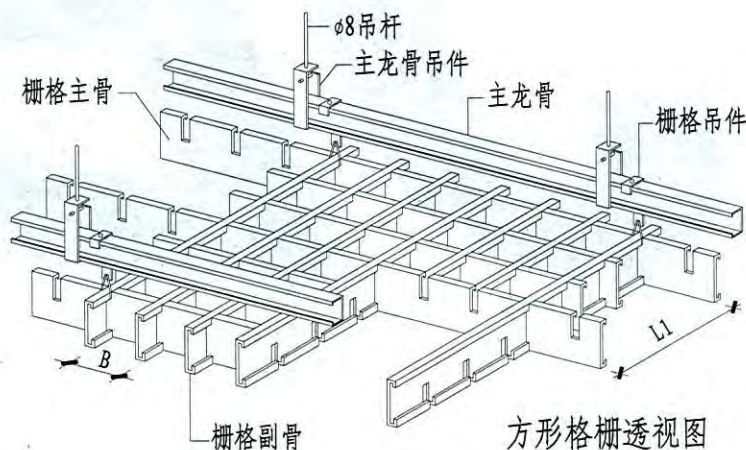
方形格栅吊顶（一）
