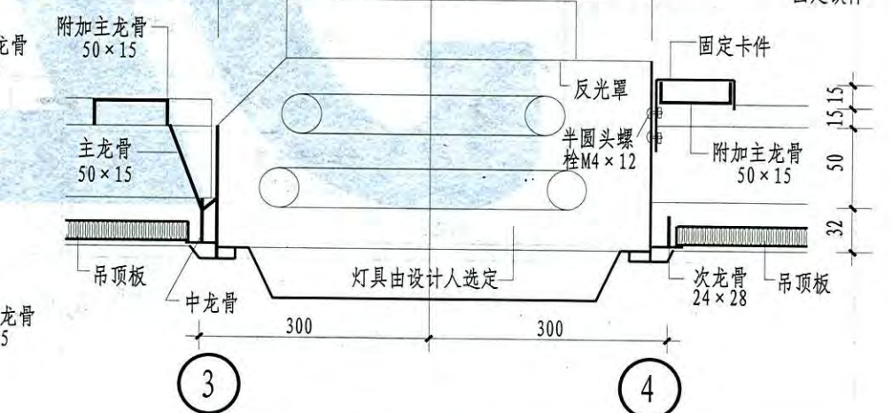
T型龙骨吊顶灯具安装
