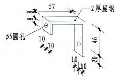
C 扁钢卡件
