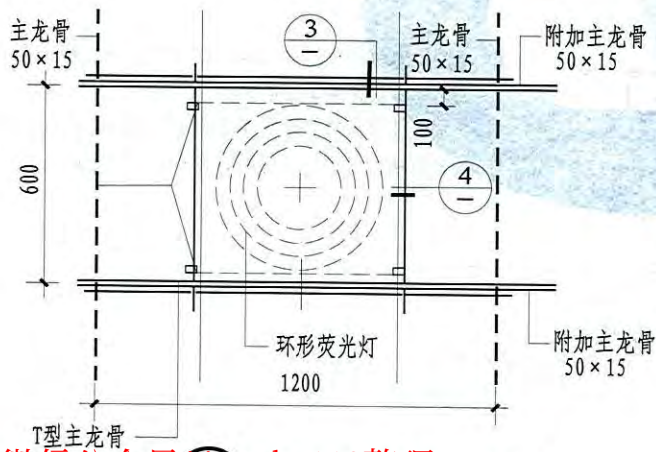
B 嵌顶灯具安装平面示意
