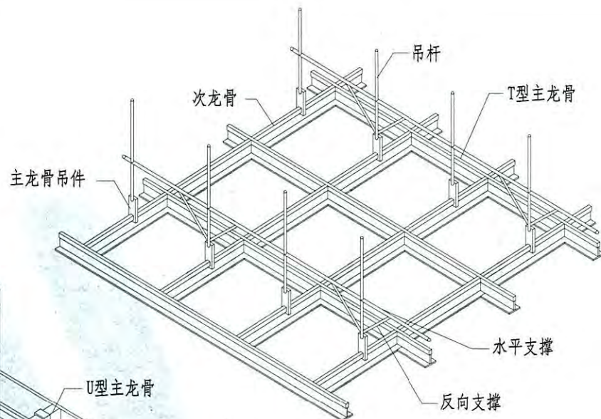
单层龙骨吊顶示意图
