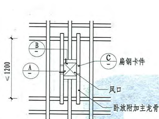
1 (风口切断次、小龙骨)
