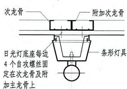
(C) (灯具重量 ≤ 4kg)
