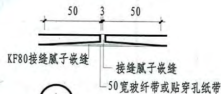
U型龙骨吊顶详图(三)
