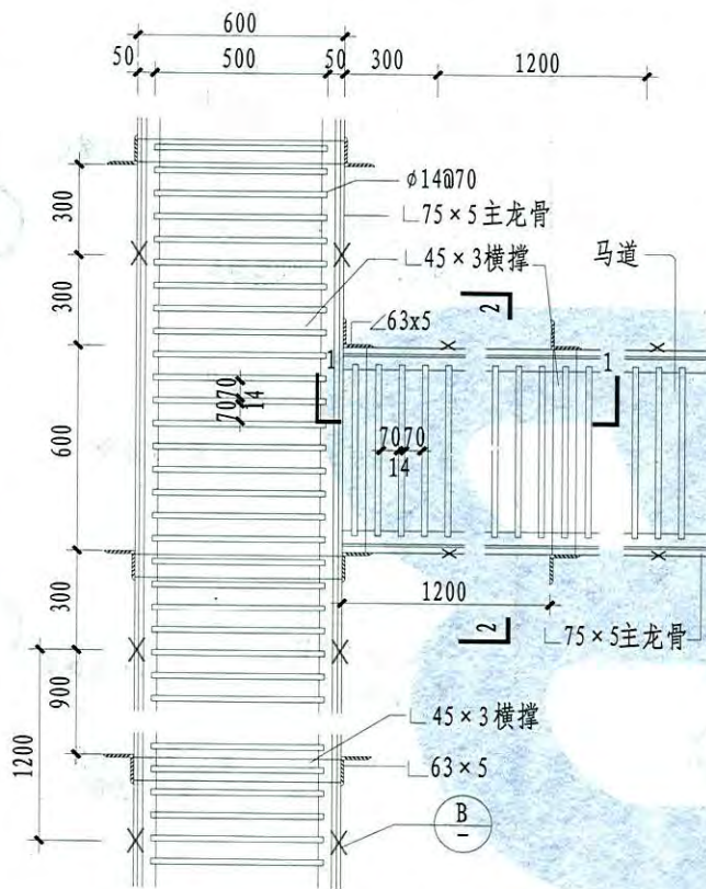
1 马道平面
